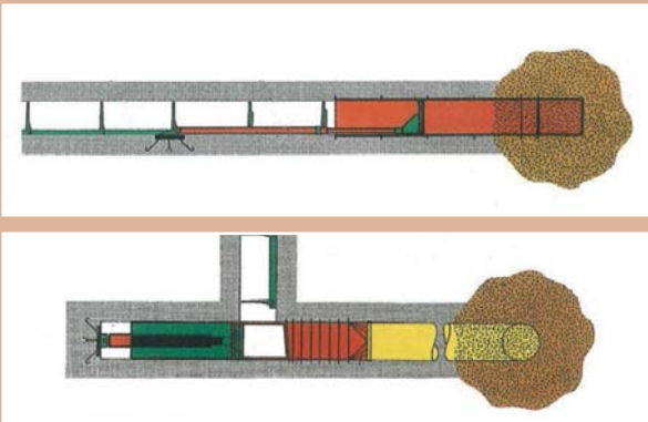
GRAFISCHE DARSTELLUNG DRUCKENTMISTUNG Standard (oben) Superpress (unten)
